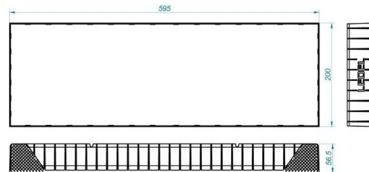
Рисунок 1а Светильник «L-school 16/Em »
