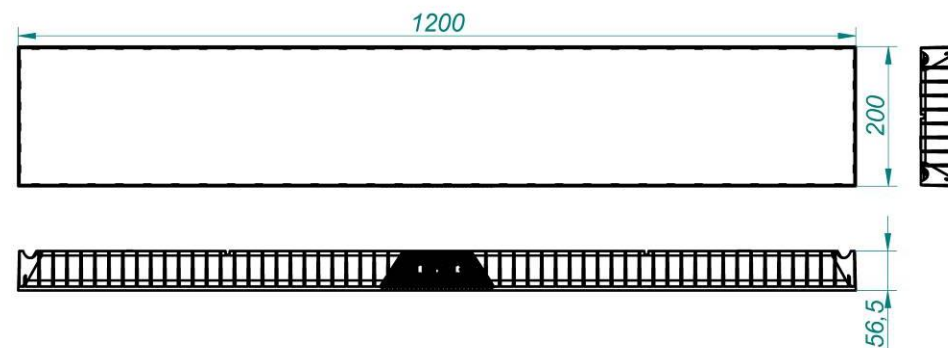
Рисунок 1б Светильник « L-school 32/Em, L-school 55/Em»
